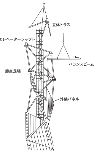
立体トラス及び外装パネル施工要領図
